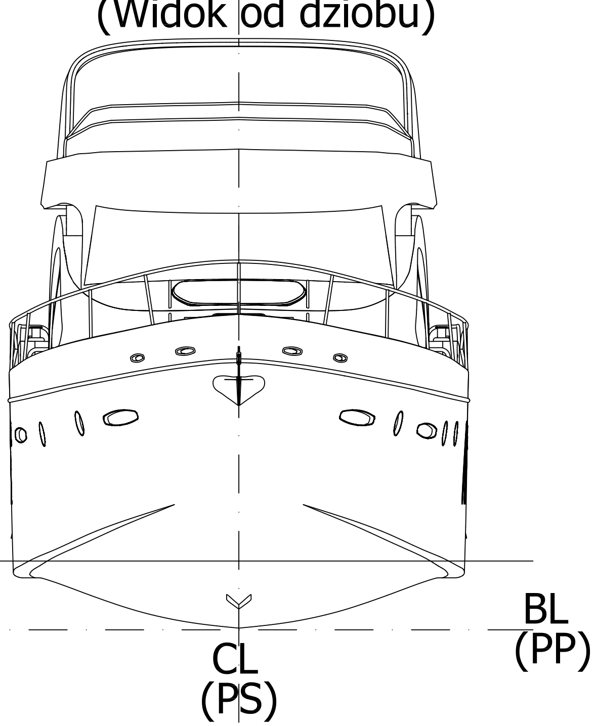
Bow view (Widok od dziobu)
