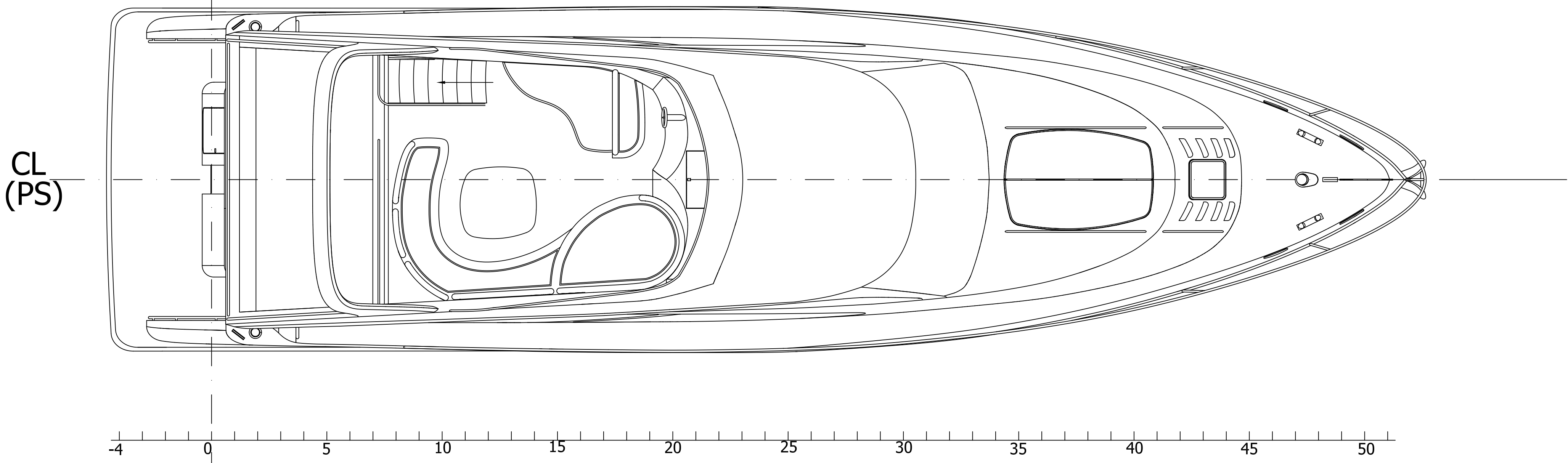
View on Main Deck (Widok na Pokład Główny)
