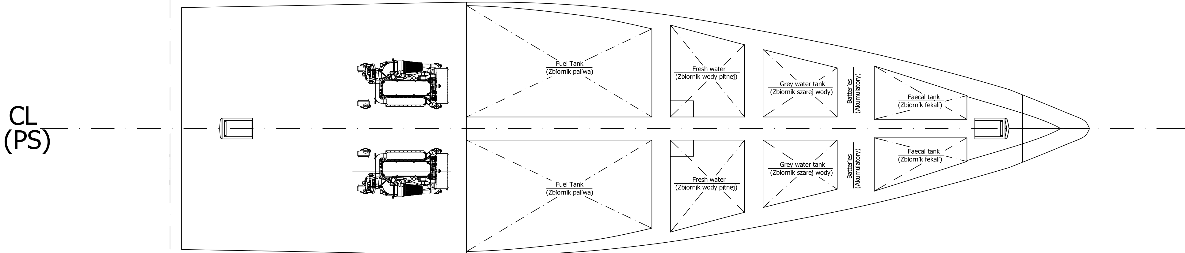
Tank plan (Plan zbiorników)
